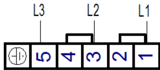
230 V 3 Ph
